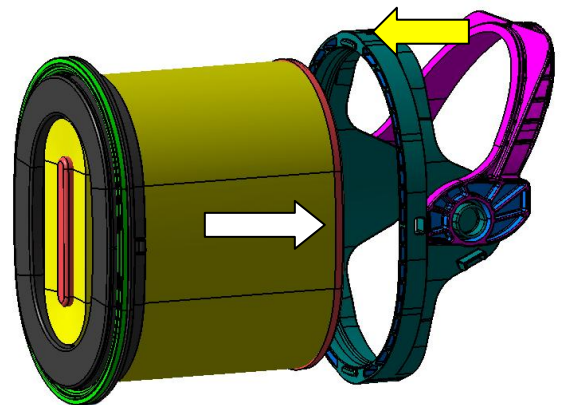
Fig. 6 Étrier de serrage IQORON tailles 10 - 14
