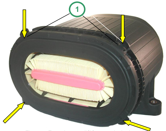
Fig. 4 Encoches sur l'élément principal
