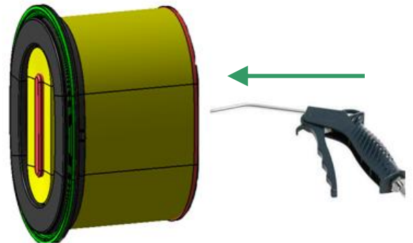
Рис. 3 Чистка основного фильтроэлемента IQORON S
