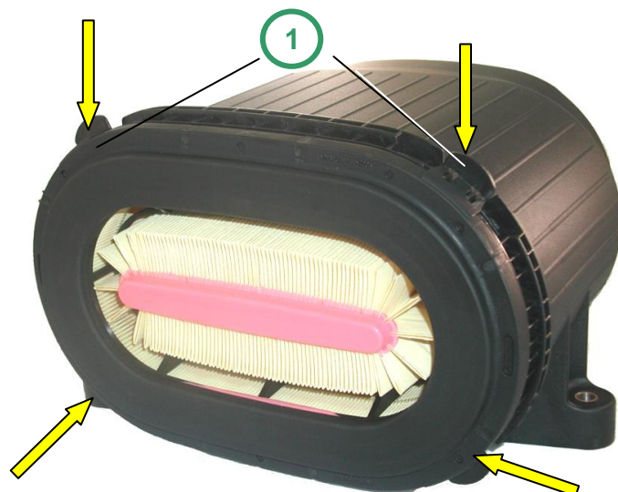
Рис. 4 Метки на основном фильтрующем элементе
