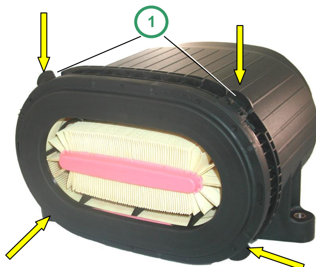
Рис. 4 Метки на основном фильтрующем элементе
