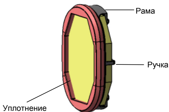
Рис. 5 Вспомогательный фильтрующий элемент
