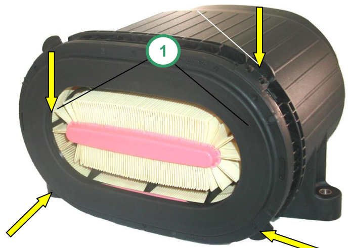
Fig. 4 Muecas en el elemento filtrante principal
